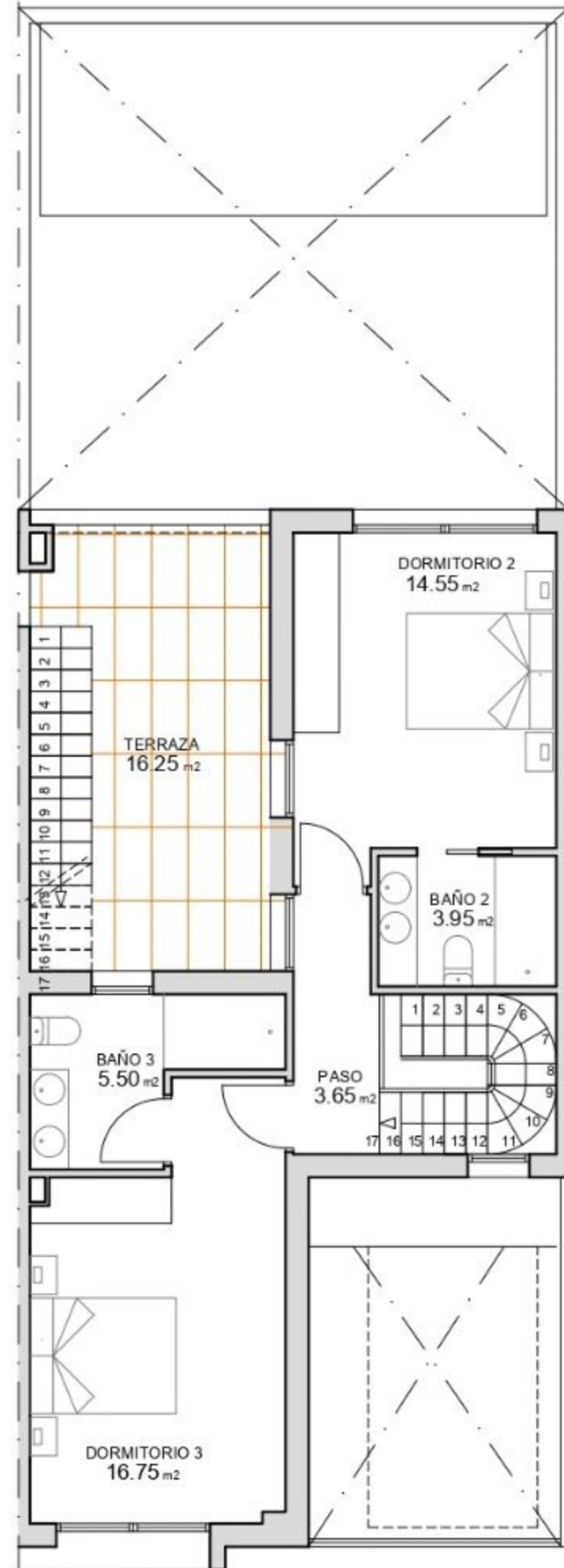
PLANTA PRIMERA
